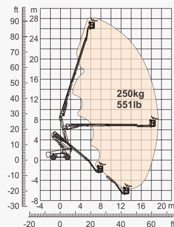
Bewegingsbereik
